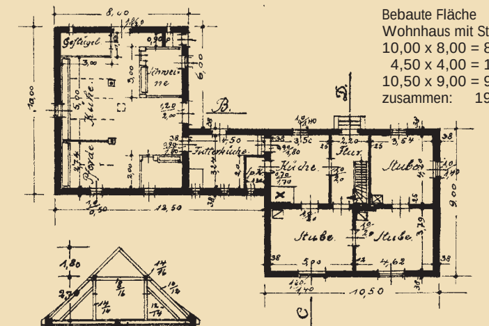
Grundriss einer Siedlerstelle, Wohnhaus mit Stall für 30 Morgen der Ostpreussischen Landgesellschaft mbH (ab 1906)
