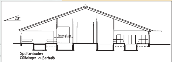
Liegeboxenlaufstall für 64 Milchkühe mit Erweiterungsmöglichkeit in Niedersachsen
